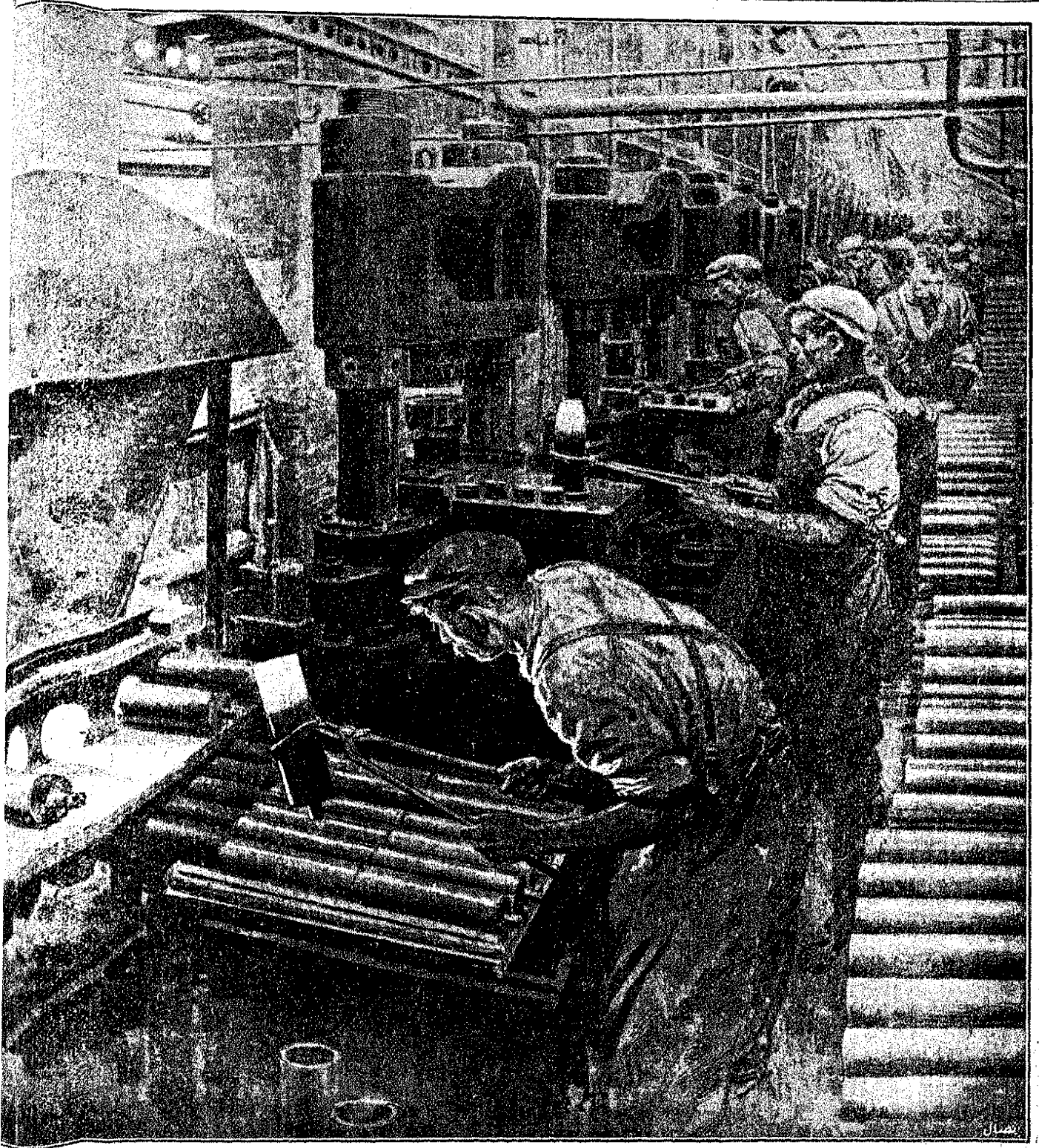
تمثل هذه الصورة عمال النخيرة في معمل فيكرس الانكليزي المشهور قترى فيها العمال يصنعون القنابل فالعامل الاول يجيئ الاسطوانة في انون من النار فتخرج نيشاء الطرفه الحرارة فيرفها بملقط على نحو ما ترى في الصورة وبناولها الى رقيقه وهذا يدخل طرف الاسطوانة في مكبس هيدروليكي فيضغط الطرف المحمي فيضيق تدريجياً حتى يصير في شكل مثل شكل قوالب السكر ثم يناوله الى رقيقه فيضمه في مكبس هيدروليكي ثان ليضيق طرف الاسطوانة ايضاً وهم جراً الى ان يتم صنع القنبلة وترى وراء العمال عدداً كبيراً من القنابل.
